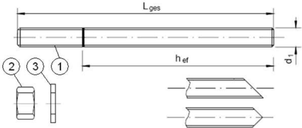
Standardgewindestange mit markierter Setztiefe
